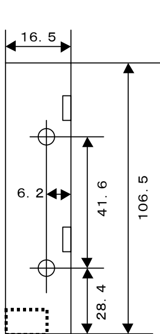
側面図 Side figure
