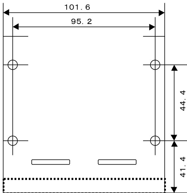
底面図 Base figure
